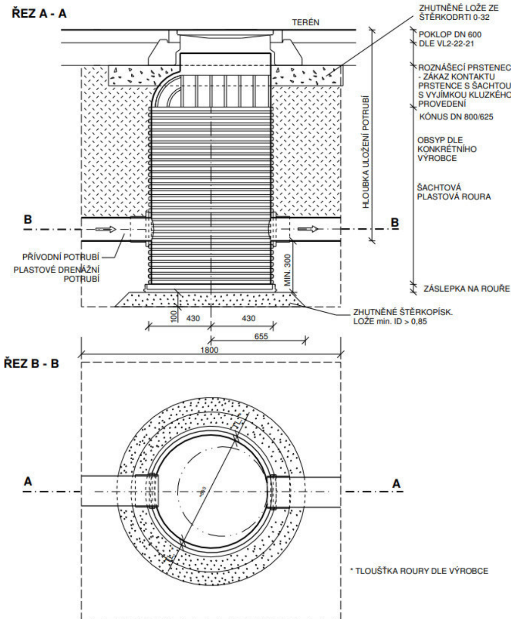
Obrázek 1 Detail drnážní šachty
