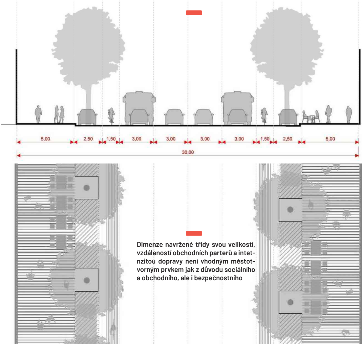
Řez uličním profilem městské třídy s MHD a s parkovacím pásem
